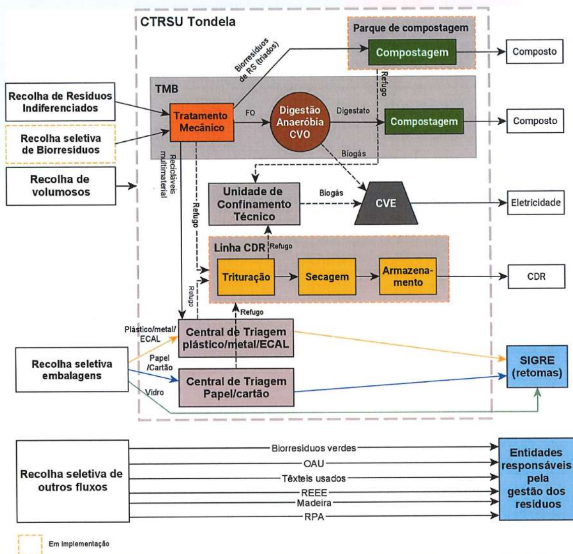
Figura 2 – Esquema ilustrativo do funcionamento do modelo técnico de gestão de RU no território da EG. 1
