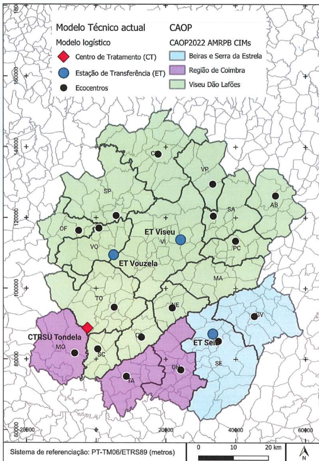
Figura 3 – Modelo logístico do SGRU.
