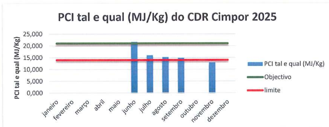
Gráfico 13 – PCI do CDR enviado para a CIMPOR
