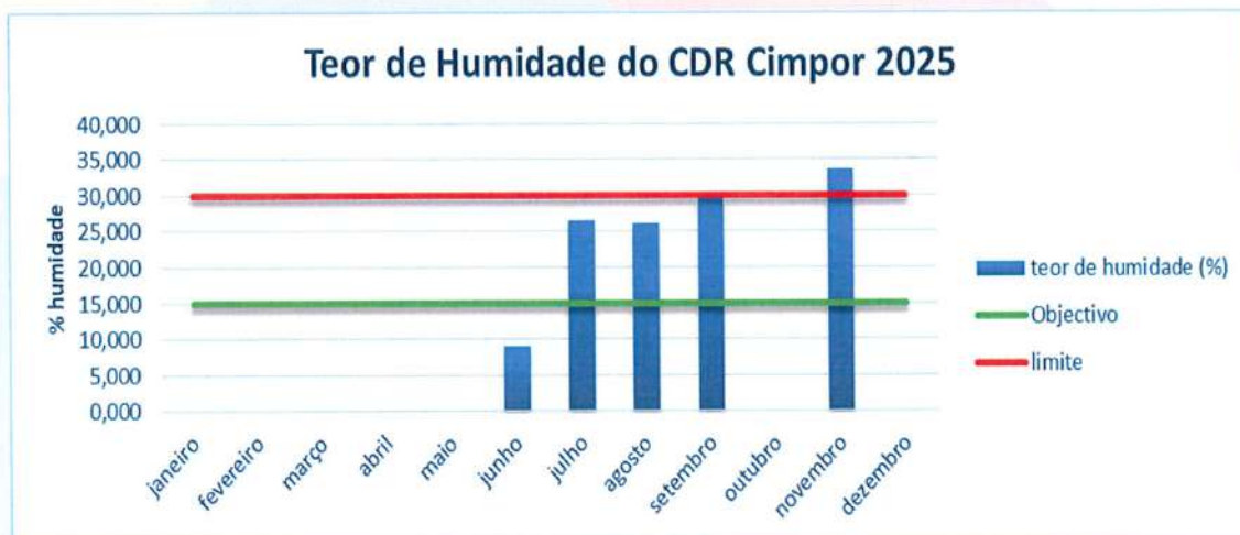
Gráfico 16 – Teor de humidade do CDR CIMPOR
