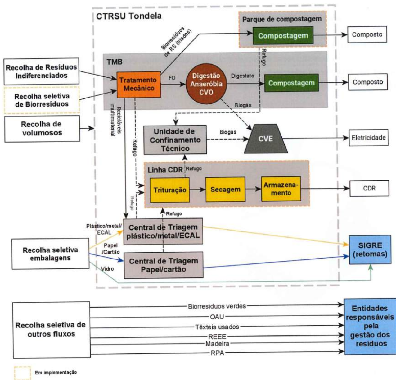
Figura 7 – Esquema ilustrativo do funcionamento do modelo técnico de gestão de RU no território da EG¹.
